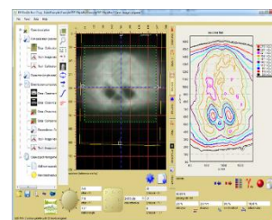
Logiciel FilmQA-Pro
